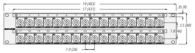
322U-BJRU 32ea 75Ω BNC-BNC Jacks
